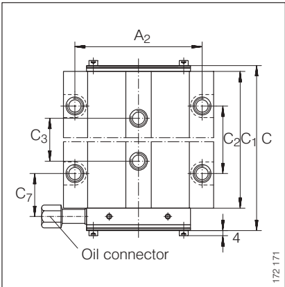
RUKS..D S
