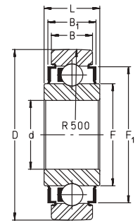
LR..RRU
