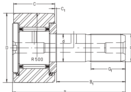
KR
