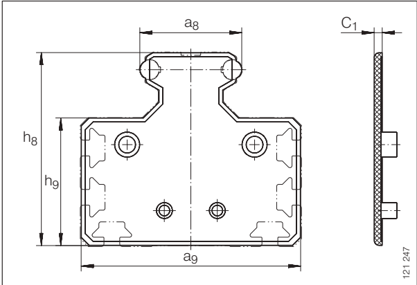
KA LFS..M
