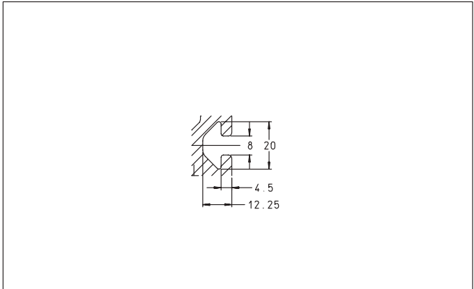
T-grooves
