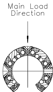
KSO, KSO..PP
