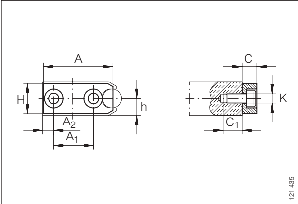
ANS LFS..FH
