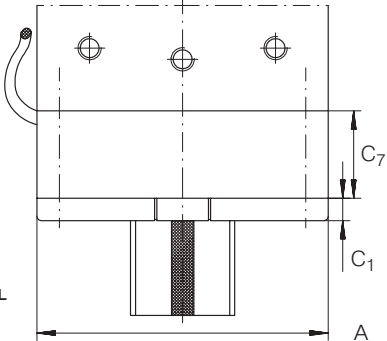
ABTKO LFKL
