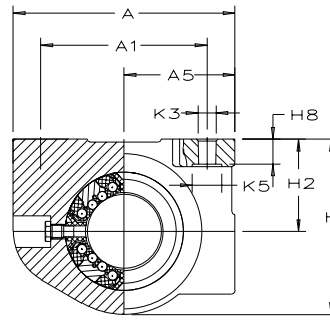
KGSAG..PP
