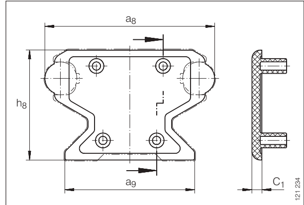
KA LFS..C
