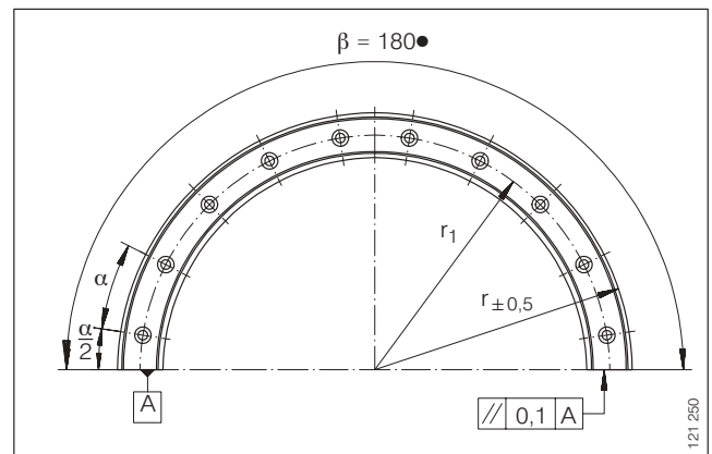
LFS..R../180
