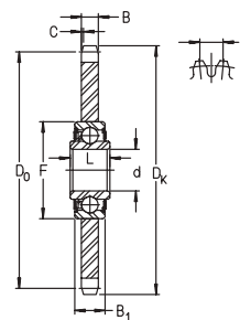
KSR..LO
