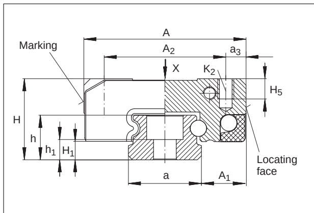
KUME 9, KUME 12
