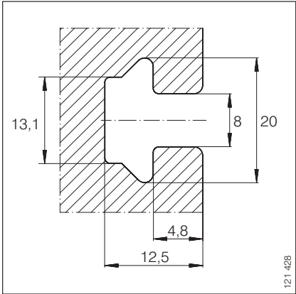
T-grooves
