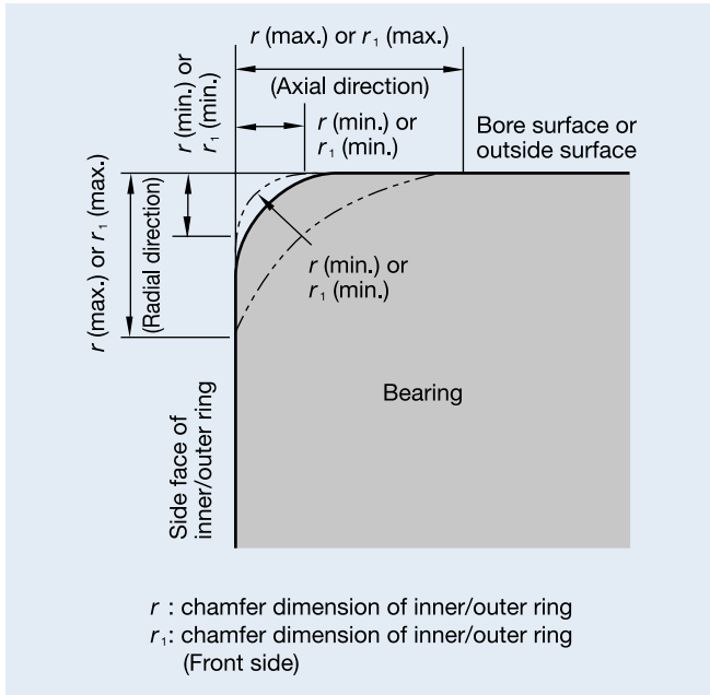
Fig. 8.2 Chamfer Dimension
