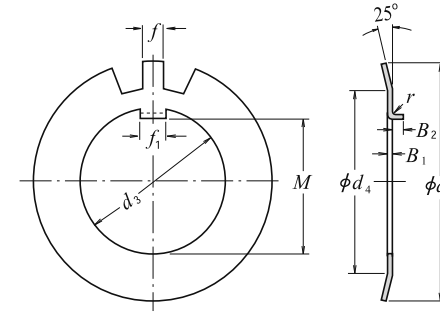
Bükülmüş Tırnak
