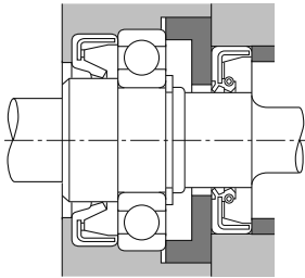
Şekil 11.8 Yağ Keçesi Uygulaması Örneği
