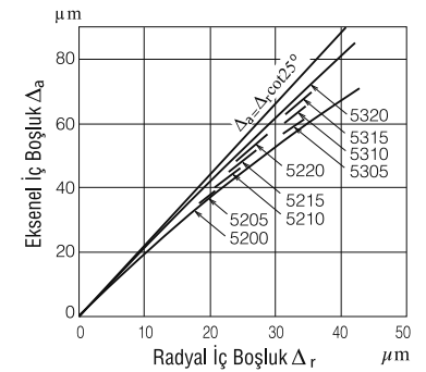
Şekil 15.8 Çift Sıralı Eğik Bilyalı Rulmanlarda \Delta_r ve \Delta_a (52, 53 Serileri)
