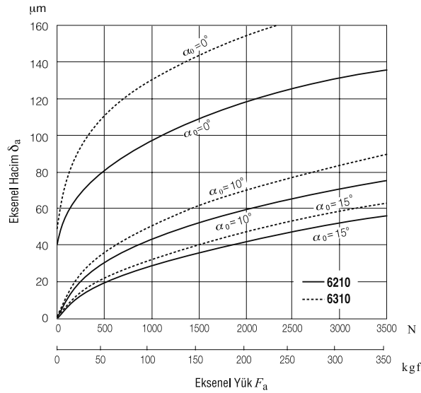
Şekil 15.2 Sabit Bilyalı Rulmanların Eksenel Yükü ve Eksenel Yer Değiştirmesi
