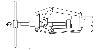
Şekil 14.14 Çekme Aleti Kullanılarak İç Bileziğin Sökülmesi (2)
