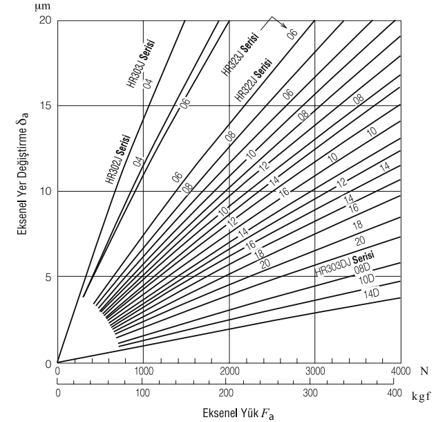
Şekil 15.4 Konik Makaralı Rulmanların Eksenel Yükü ve Eksenel Yer Değiştirmesi
