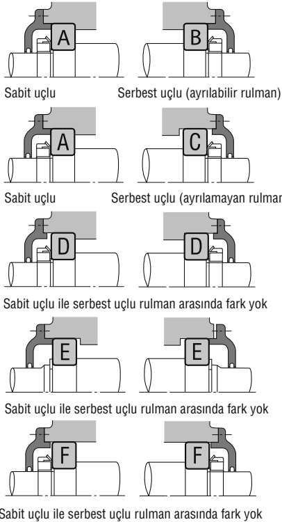
Şekil 4.1 Rulman Montaj Düzenleri ve Rulman Tipleri
