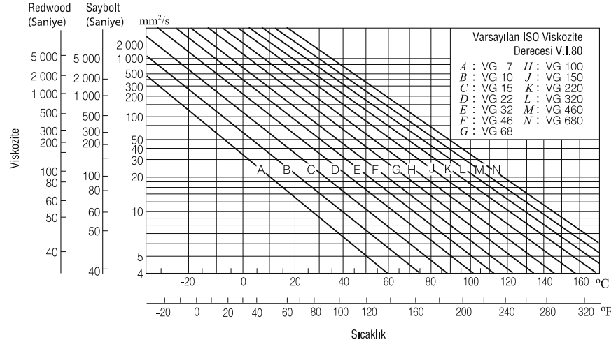
Şekil 12.11 Sıcaklık-Viskozite Tablosu
