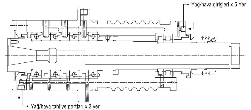
Şekil 12.10 Yağ/Hava Yağlaması
