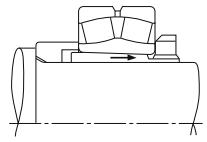
Şekil 14.4 Adaptörlü Montaj
