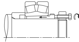
Şekil 14.5 Çekme Maşonlu Montaj
