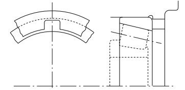
Şekil 14.11 Sökme Çentikleri
