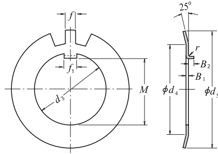
Bükülmüş Tırnak
