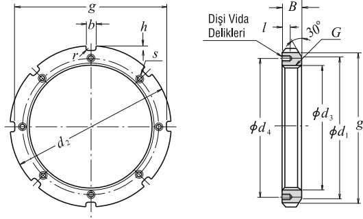
Stoperli Somun
