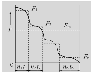
Şekil 5.7 Artımlı Yük Değişimi
