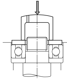
Şekil 14.2 İç ve Dış Bileziklerin Eşzamanlı Presle Geçmesi
