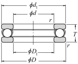
Düz Yataklı
