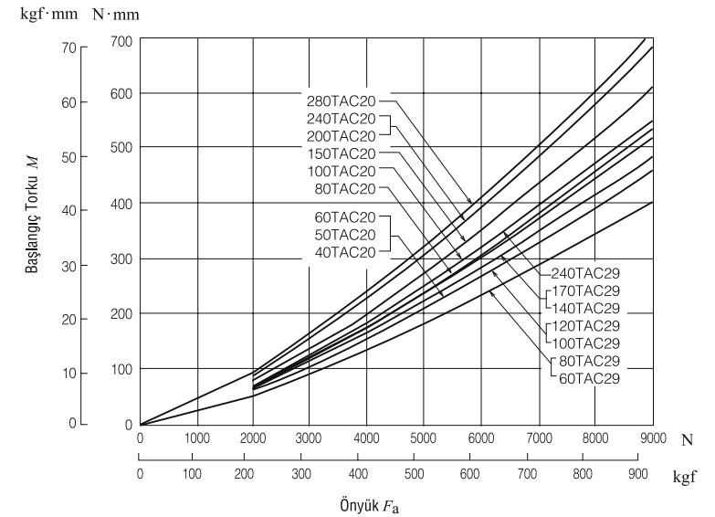
Şekil 15.12 Çift Yönlü Eğik Eksenel Bilyalı Rulmanların Önyükü ve Başlangıç Torku
