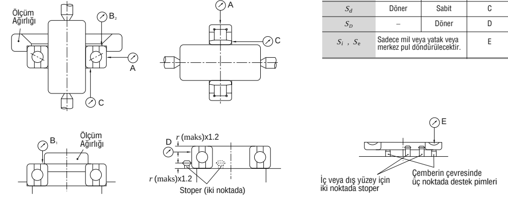
Şekil 8.1 Çalışma Hassasiyeti için Ölçüm Yöntemleri (özet)
