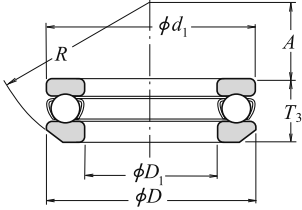
Oynak Yataklı
