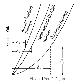
Şekil 10.6 Rijiditenin ve Ön Yükleme Yöntemlerinin Karşılaştırılması
