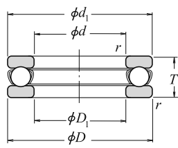
Düz Yataklı
