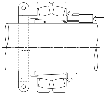
Şekil 14.18 Stoper ve Eksenel Basıncı ile Adaptörün Sökülmesi
