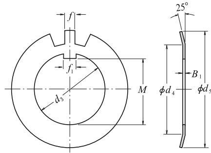
Düz Tırnak
