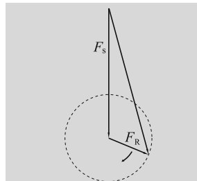
Şekil 5.10 Döner Yük ve Sabit Yük
