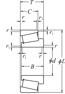
Şekil 7.2 Konik Makaralı Rulmanlar
