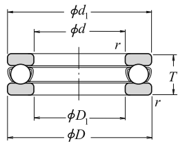
Düz Yataklı
