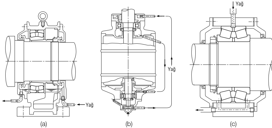
Şekil 12.7 Devirdaimli Yağlama
