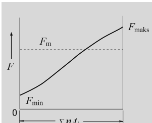
Şekil 5.8 Basit Yük Dalgalanması
