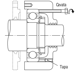
Şekil 14.10 Sökme Cıvatalarıyla Dış Bileziğin Sökülmesi
