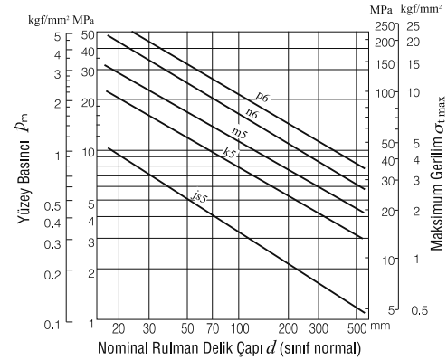
Şekil 15.5 Ortalama Sıkı Geçme Toleransı için Yüzey Basıncı p_m ve Maksimum Gerilim \sigma_{tmax}
