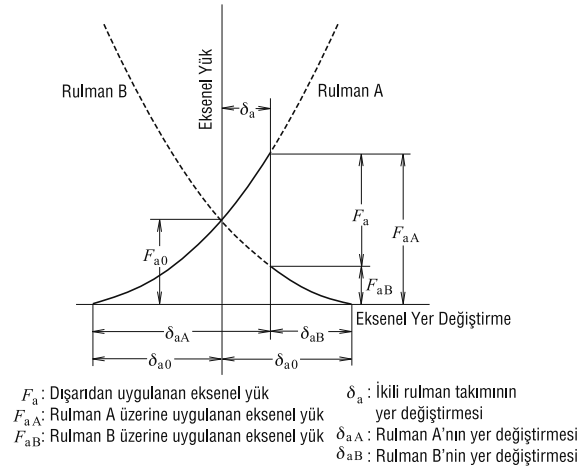
Şekil 10.4 Konum Önyükü ile Eksenel Yer Değiştirme
