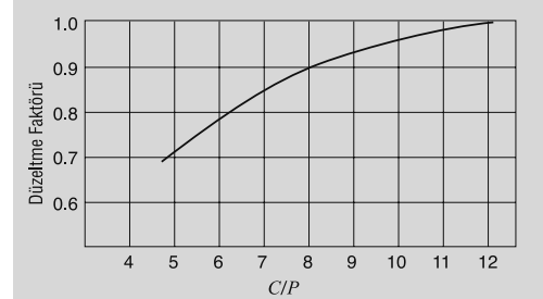
Şekil 6.1 Yük Kapasitesiyle Limit Hız Düzeltme Faktörü Değişimi
