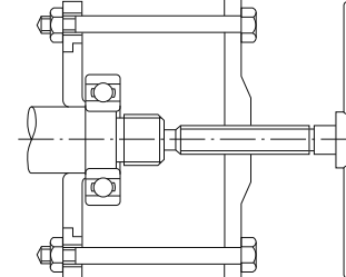
Şekil 14.13 Çekme Aleti Kullanılarak İç Bileziğin Sökülmesi (1)
