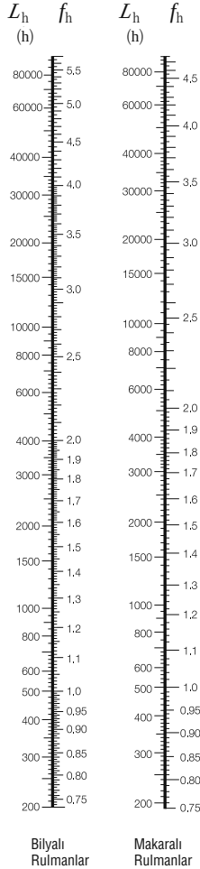
Şekil 5.4 Yorulma Ömrü Faktörü ve Yorulma Ömrü
