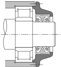
Şekil 11.9 Yağ Keçesi Uygulaması Örneği (2)
